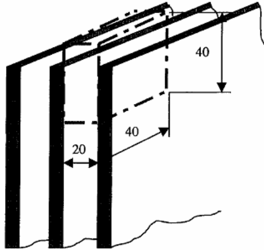
图 A3 玻璃的垂直支撑及间隔体
